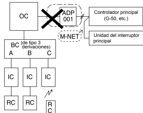
3-3. Conexión del adaptador M-NET a la unidad exterior
