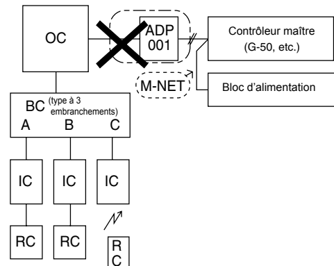
3-3. Raccordement d'un adaptateur M-NET à l'appareil extérieur
